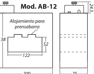
Mod. AB-12 2500 a 3000/5 5/10VA Cl. 1 PRECIO 250,00
