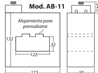
Mod. AB-11 2500 a 3000/5 5/10VA Cl. 1 PRECIO 237,50
