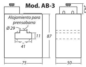
Mod. AB-3 400 a 630/5 5VA Cl. 0,5 PRECIO 143,75
