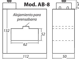
Mod. AB-8 1200 a 2000/5 5VA Cl. 1 PRECIO 206,25
