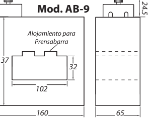
Mod. AB-9 2000/5 5VA Cl. 1 2000/5 10VA Cl. 0,5/1 PRECIO 218,75
