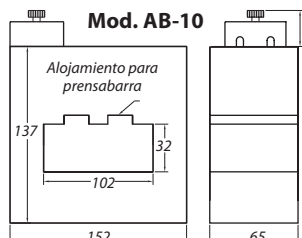
Mod. AB-10 2500 a 3000/5 5/10VA Cl. 1 PRECIO 225,00
