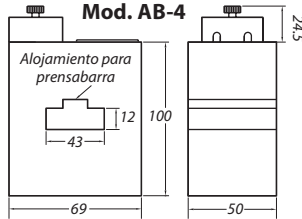
Mod. AB-4 630/5 5VA Cl. 0,5 PRECIO 150,00
