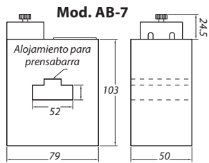
Mod. AB-7 630 a 1250/5 5VA Cl. 0,5 PRECIO 198,75
