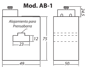
Mod. AB-1 100 a 150/5 5VA Cl. 0,5/1 160 a 200/5 5Va Cl. 1 PRECIO 110,50
