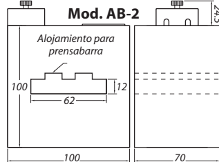
Mod. AB-2 250 a 400/5 5VA Cl. 0,5/1 500 a 600/5 10Va Cl. 1 PRECIO 136,50
