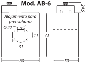
Mod. AB-6 250/5 5VA Cl. 0,5 PRECIO 187,50
