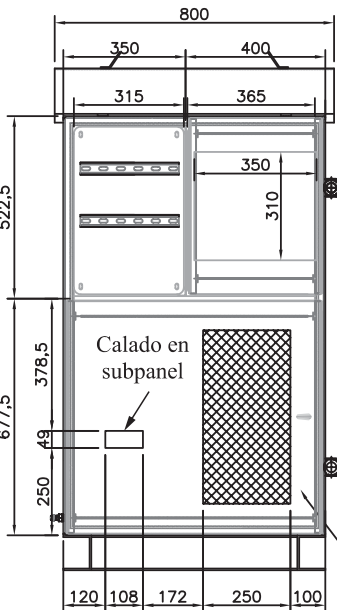
Vista frontal puertas subpaneles
