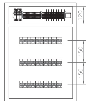
Vista frontal Distribución interna
