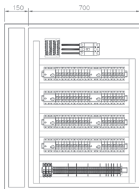
Vista frontal Distribución interna
