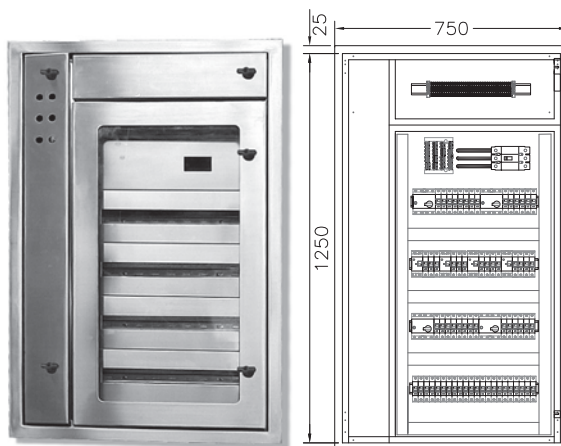
Vista frontal Distribución interna
