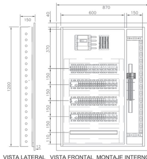
VISTA LATERAL VISTA FRONTAL MONTAJE INTERNO
